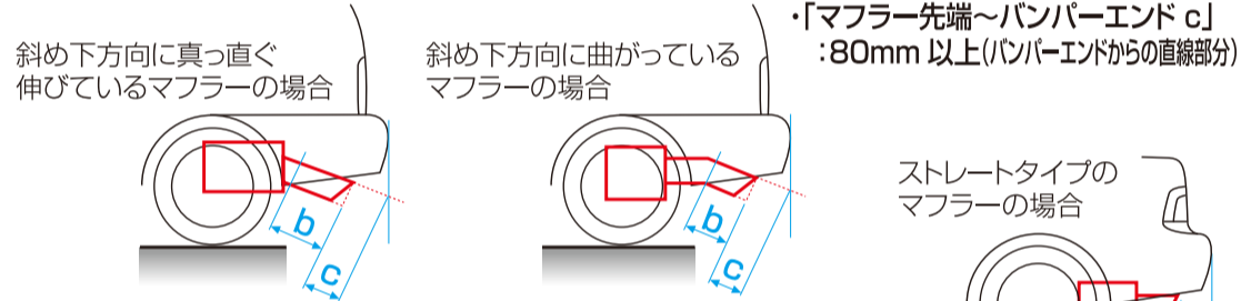
(図 4) 純正マフラーと車体(リアバンパー)のすき間
