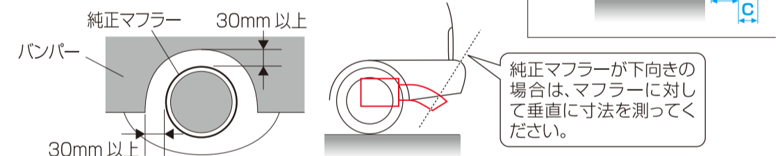
(図 4) 純正マフラーと車体(リアバンパー)のすき間
