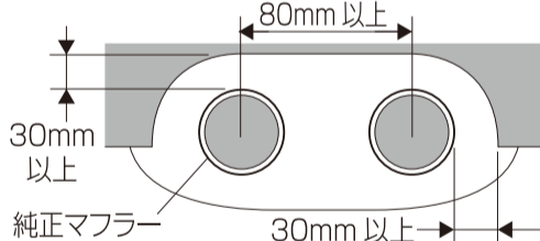
(図 5) デュアルマフラー
