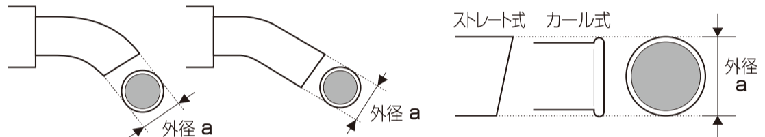
(図 3) 純正マフラーの長さ
