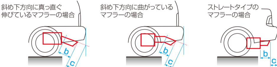
(図3) 純正マフラーと車体(リアバンパー)のすき間
